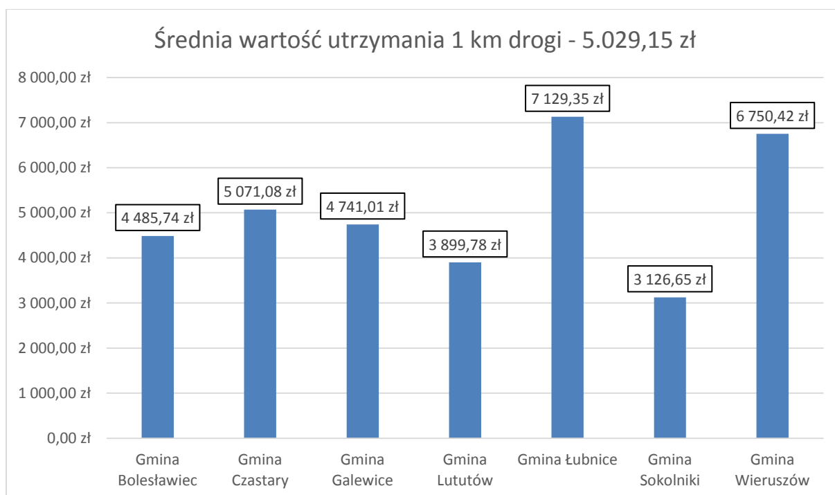
Wykres nr 22 Średnia wartość bieżącego utrzymania 1 km drogi z podziałem na gminy
